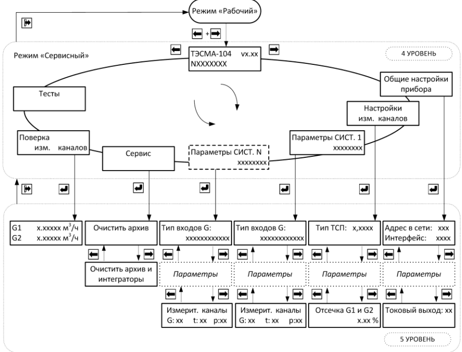
Рис. 9.3 Режим «Сервисный»
